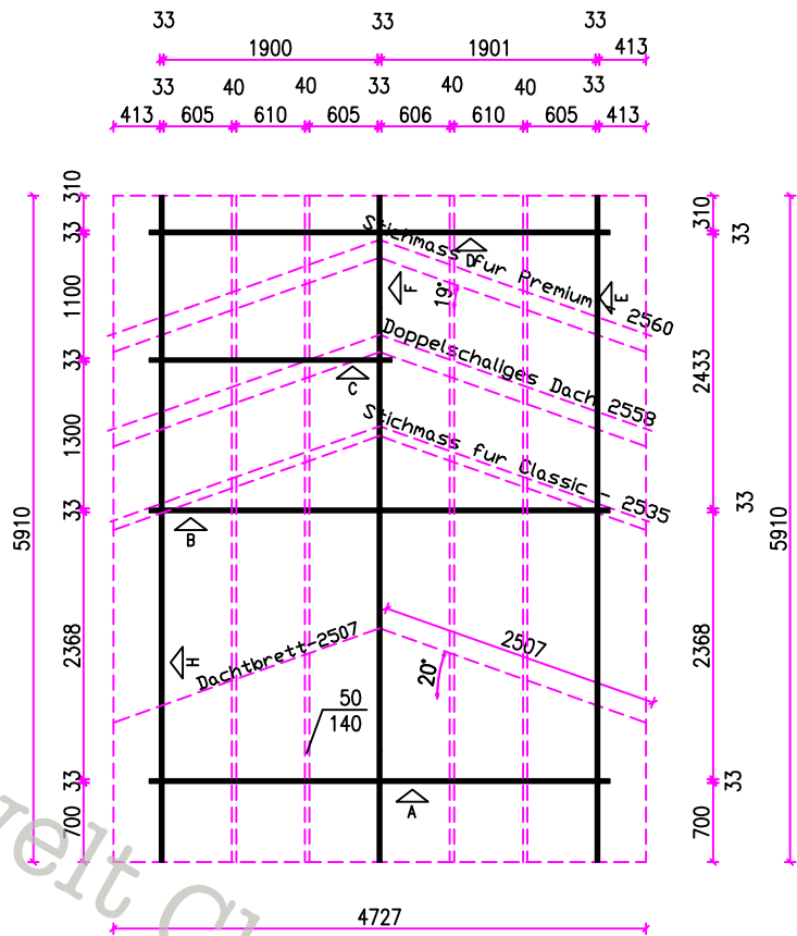
DACHPLAN
