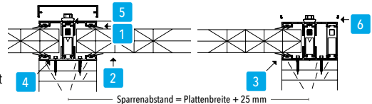
Verbindungsprofil
