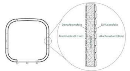
127 mm starke isolierte Dach- und Seitenwände
