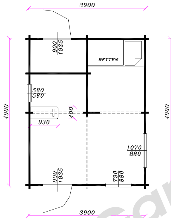
GRUNDRISS
