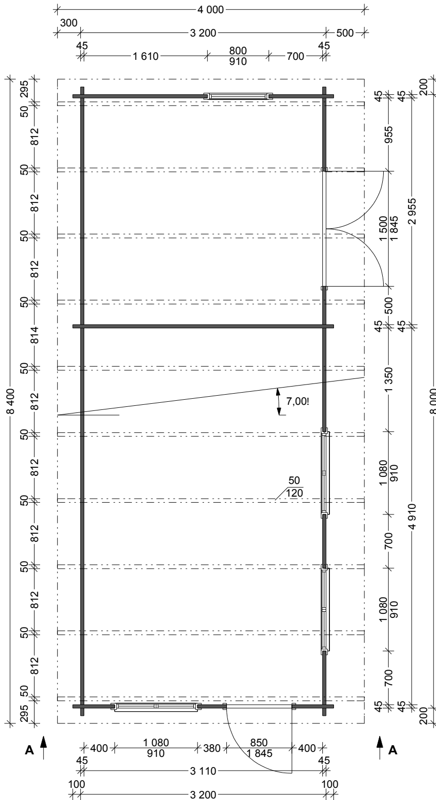
Tür, Fenster - Bauwischer kotiert
