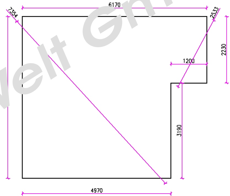
FUNDAMENTPLATTE
